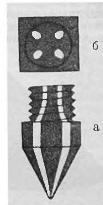
Фиг. 4. а) Винтовой шипъ съ 4 стальными жилами; б) Поперечн. разрѣзъ его.
